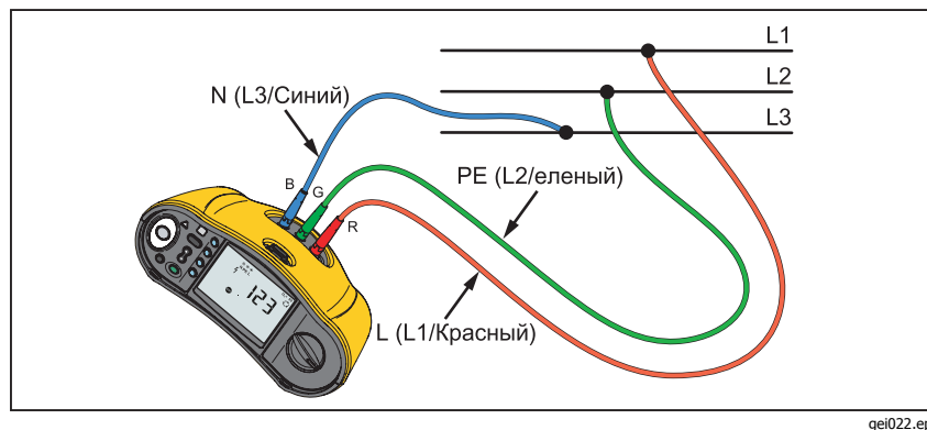
Рис. 10. Подключение для проверки чередования фаз
