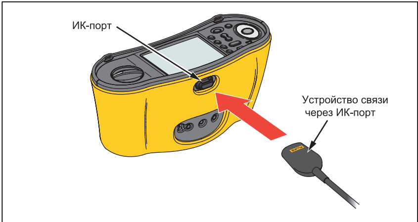
Рис. 16. Подключение последовательного ИК-кабеля
