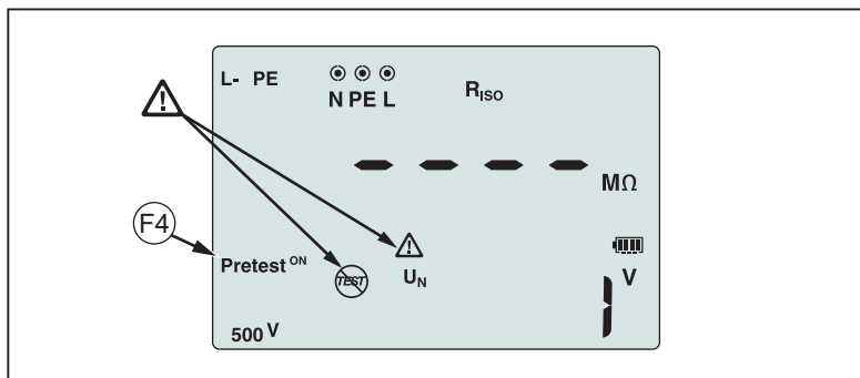
Рис. 5. Экран функции предварительного тестирования безопасности
