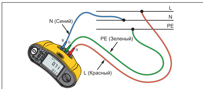
Рис. 4. Соединение для функции предварительного тестирования безопасности
