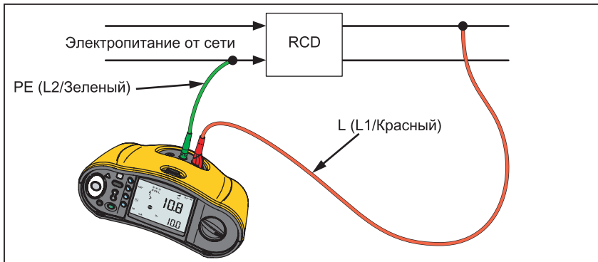
Рис. 8. Подключение для проверки УЗО на электрических системах IT
