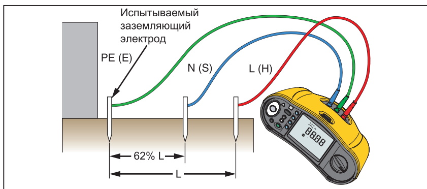
Рис. 12. Соединение для проверки сопротивления заземления
