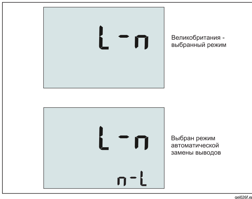
Рис. 1. Режимы переключения положения проводов
