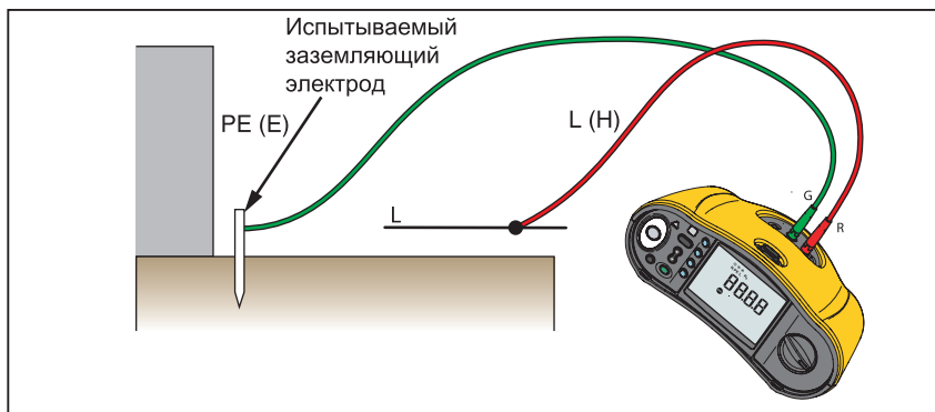
Рис. 14. 2-проводное соединение для контурной проверки сопротивления заземления (режим размыкания по высокому току)
