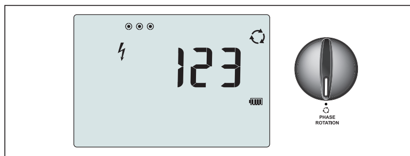
Рис. 11. Дисплей чередования фаз
