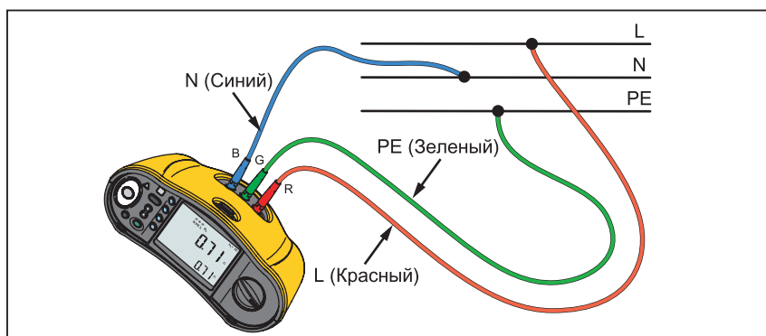
Рис. 13. 3-проводное соединение для контурной проверки сопротивления заземления (режим без размыкания)
